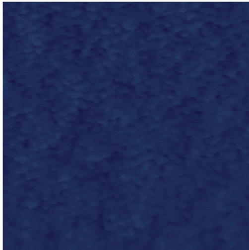
CdSe 3.0 MLs
