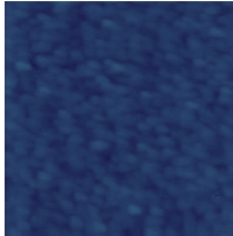
CdSe 2.7 MLs
